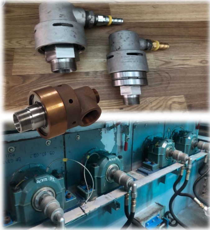
Rotary union Khớp nối xoay cho con lăn
