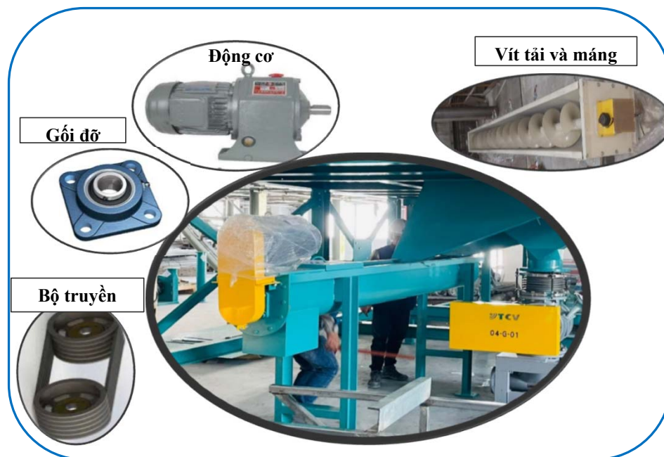
Vít tải và phụ kiện Screw conveyor & parts
